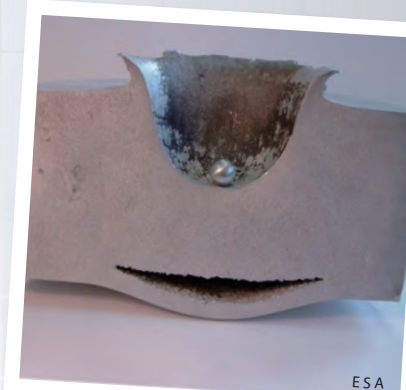
在歐洲太空總署（ESA）模擬太空垃圾的高速撞擊中，研究發現，就算是直徑1公分多的小鋼球，在20倍的音速下，也能把18公分厚如牆壁的鋼板撞出一個大凹洞。
