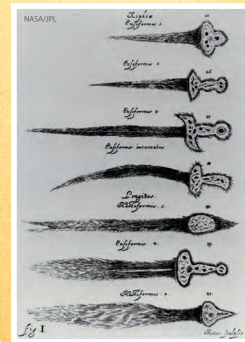
這是十七世紀天文書籍裡的圖，其中有些彗星看起來就像燃燒的劍。
